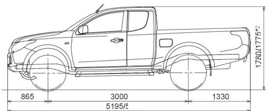
Schéma vozidla:
